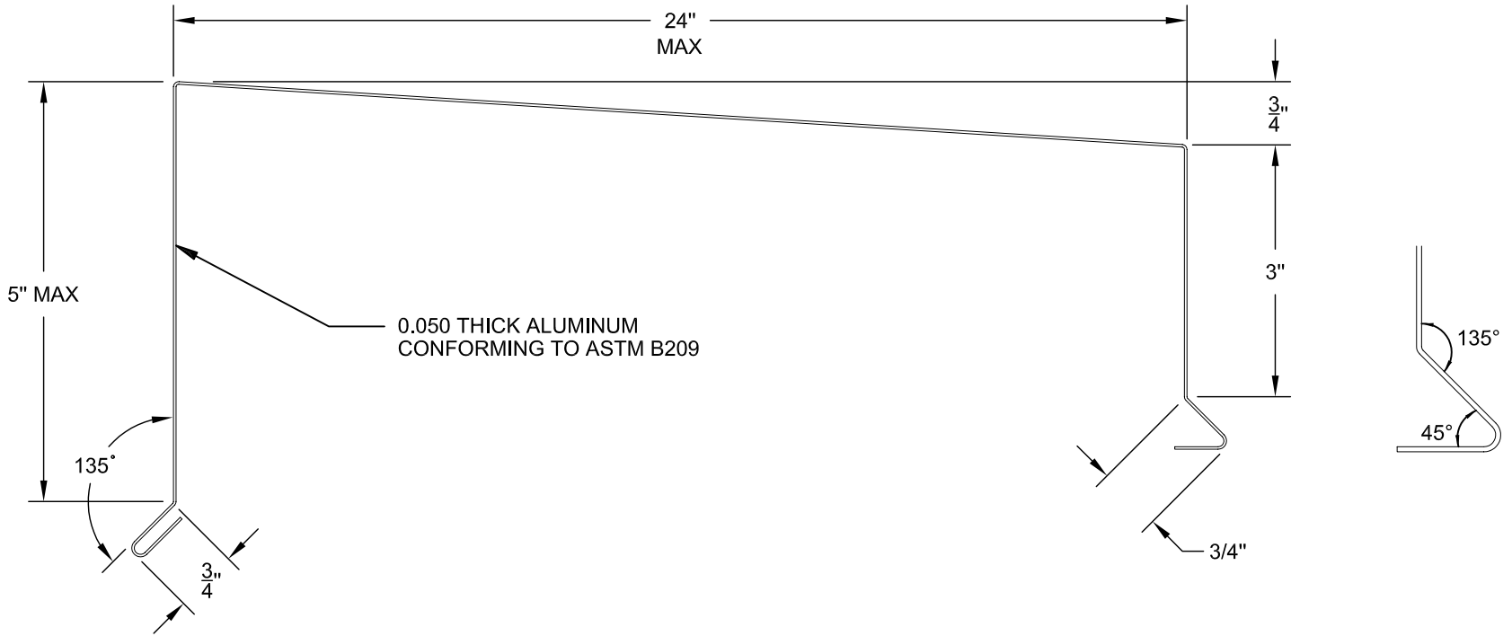
PARAPET CAP
