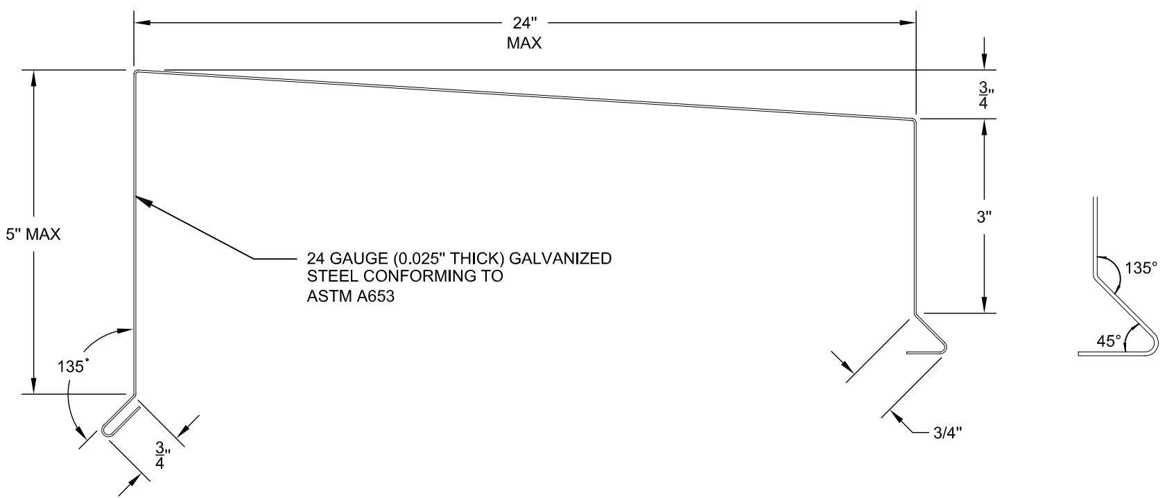
PARAPET CAP
