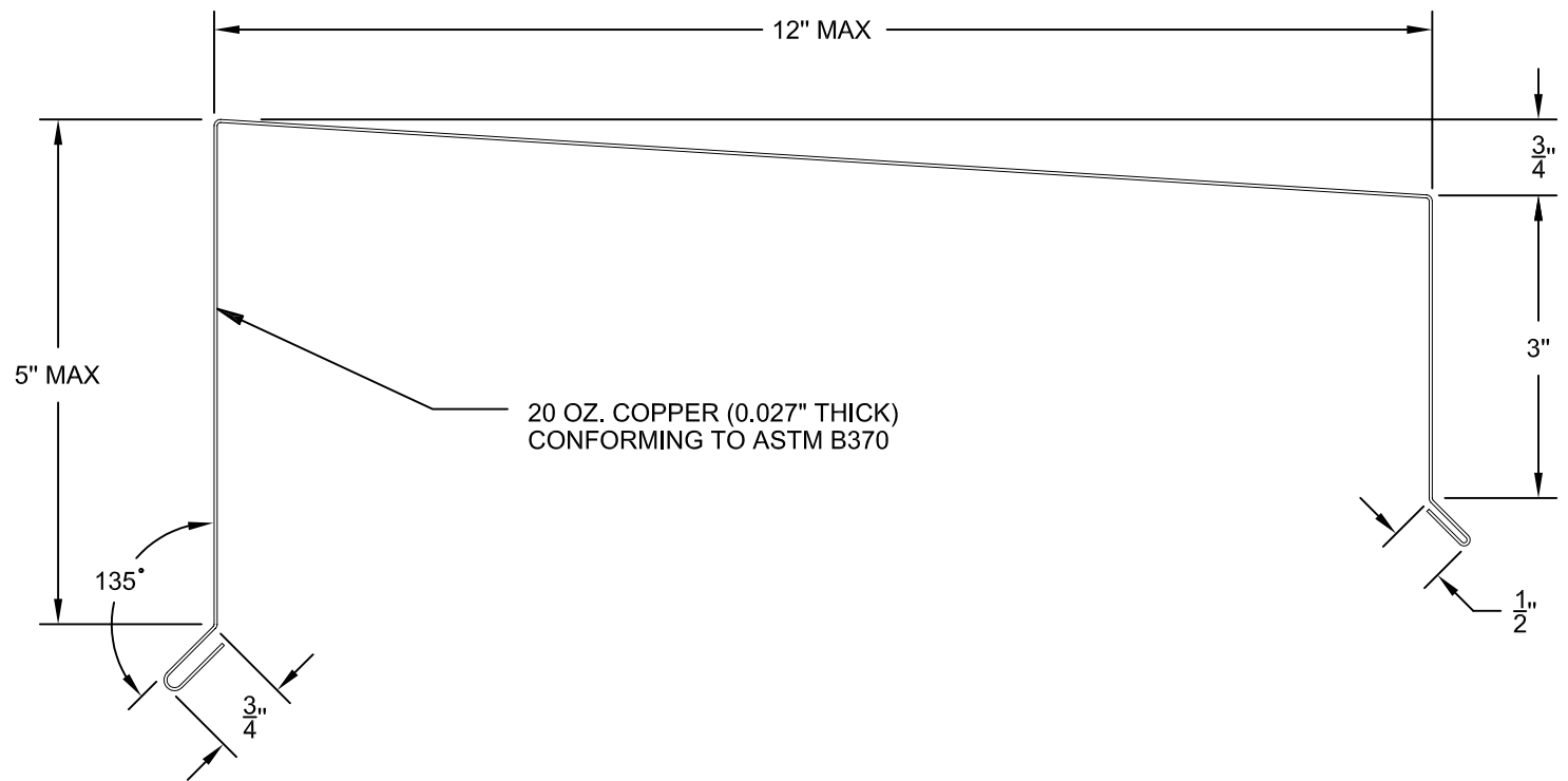
PARAPET CAP
