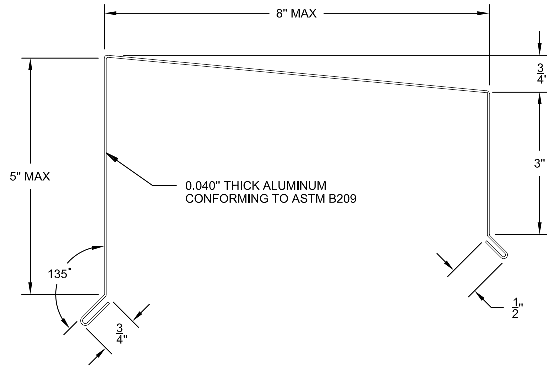
PARAPET CAP
